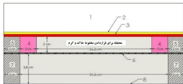
شکل ۵: ترتیب قرارگیری بخش‌های مختلف دستگاه برداشت کرم سفید. ۱- وزنه، ۲- منبع حرارتی (زرد رنگ)، ۳- صفحه آلومینیومی (قرمز)، ۴- عایق، ۵- دیواره‌های کناری چوبی، ۶- توری (چشمه ۲/۵ mm)، ۷- پایه‌های چوبی، ۸- صفحه پلکسی گلاس (پلاستیک شفاف) (Pompeo, 2017)
