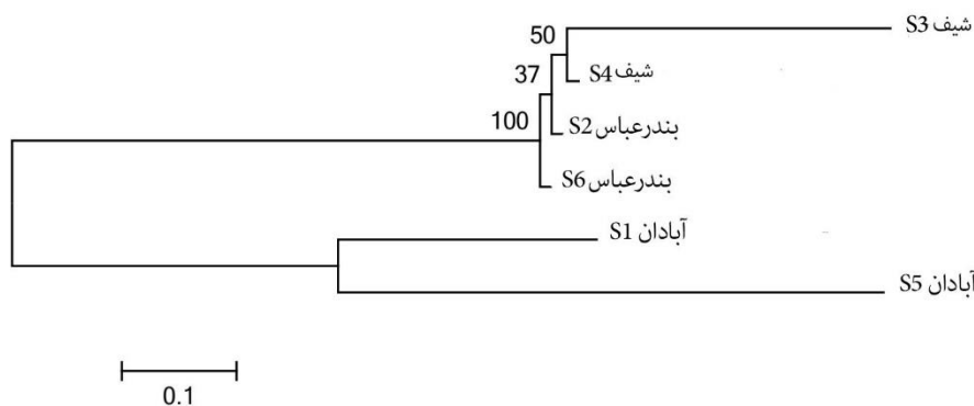
شکل ۵: درخت فیلوژنی بر اساس روش Maximum linkhood برای گونه Chirocentrus nudus در مکان‌های نمونه‌برداری با استفاده از ژن COI
